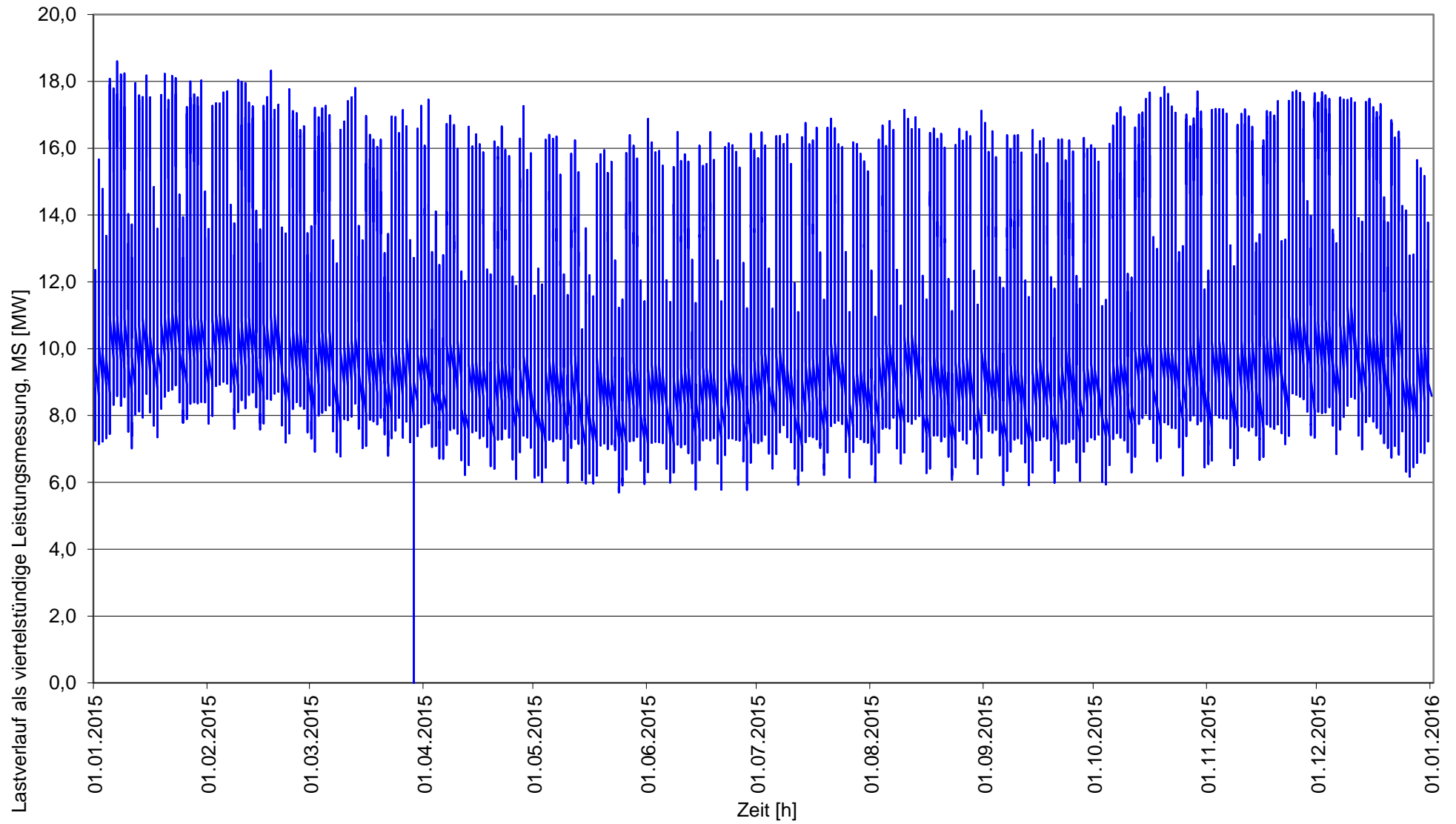
Lastverlauf als 1/4-h Leistungsmessung Mittelspannung
